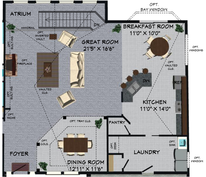
OPTIONAL ATRIUM PLAN
